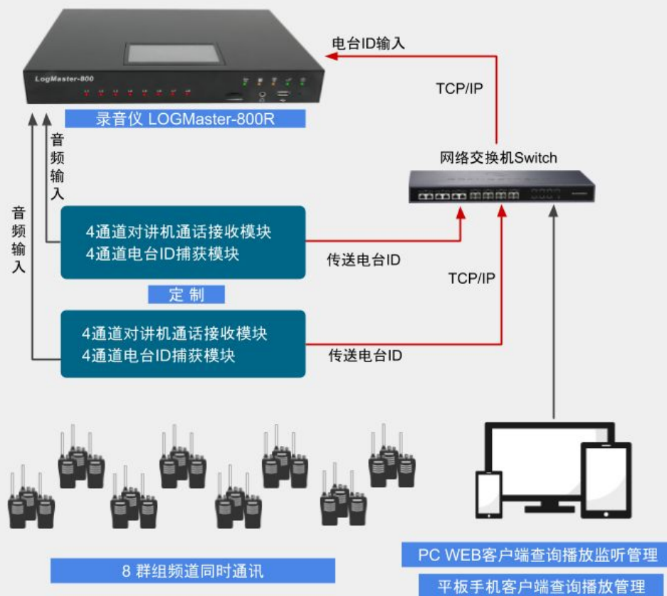
一体式录音仪 (专业电台对讲机录音专用) LOGMaster-800R
